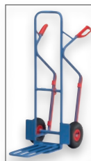
Klappbare Stahlrohrschaufel L 500 x B 250 mm
